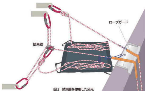
図2 結束器を使用した吊元
